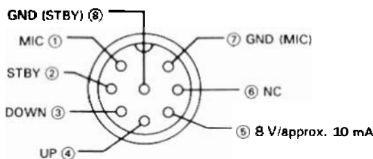
Connecteur Micro (Vue de face)
