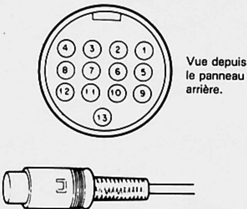
Fiche standard DIN, 13 broches (E07-1351-05)
