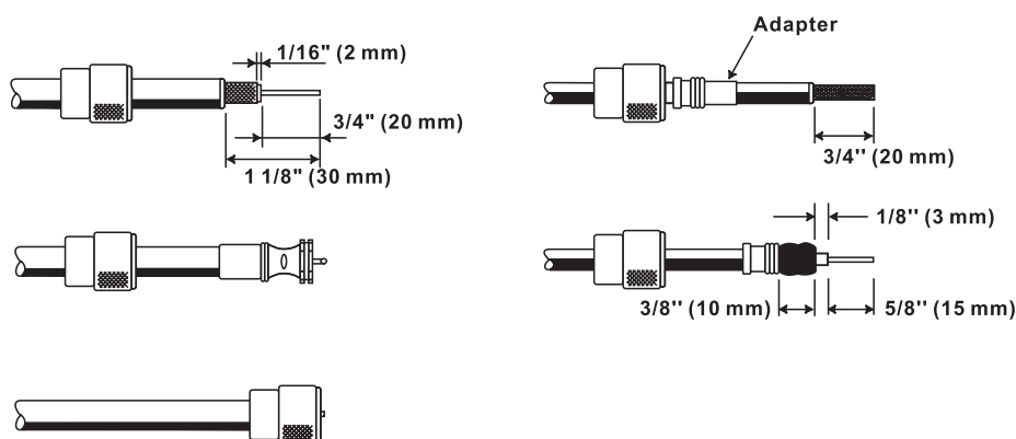
INSTALLATION TYPE DES PL-259
