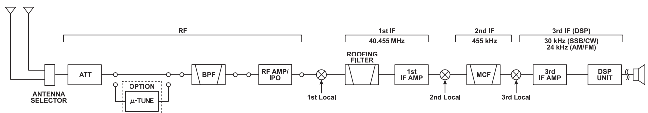
SCHEMA FONCTIONNEL DES ÉTAGES D'ENTRÉE
